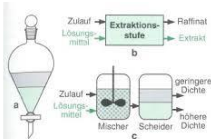
8.3 Flüssig-Flüssig-Extraktion; a Scheidetrichter für diskontinuierliche Extraktion, b Schema einer kontinuierlich betriebenen Extraktionsstufe, c Skizze einer Mischer-Scheider-Einheit für kontinuierlichen Betrieb.
