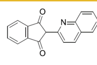
solvent yellow 33 (gelb)
