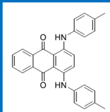
solvent green 3 (blau)
