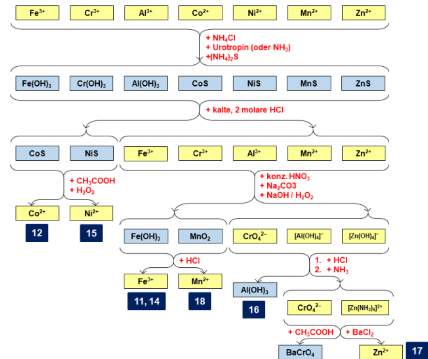
Abbildung 9: Übersicht über den Trennungsgang der Kationen der (\text{NH}_4)_2\text{S} -Urotropin-Gruppe.
